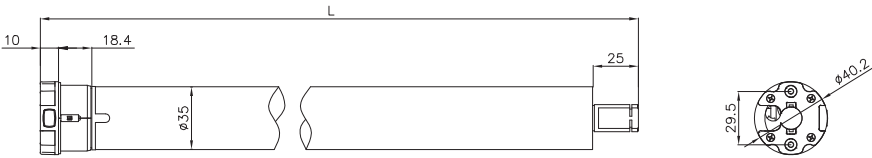
Motor dimensions / 电机外形尺寸图
