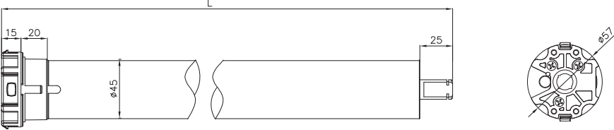
Motor dimensions / 电机外形尺寸图
