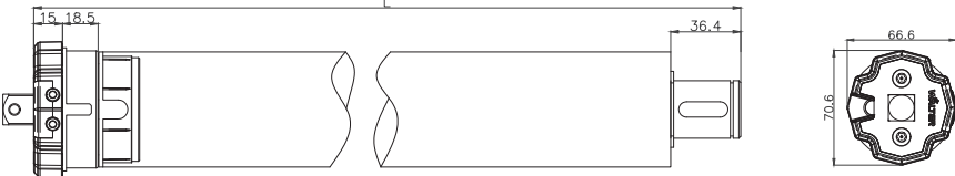
Motor dimensions / 电机外形尺寸图
