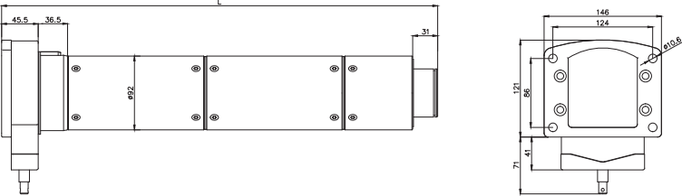
Motor dimensions / 电机外形尺寸图
